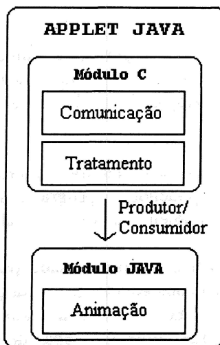
Figura 3 – Estrutura do Monitor de Execução
