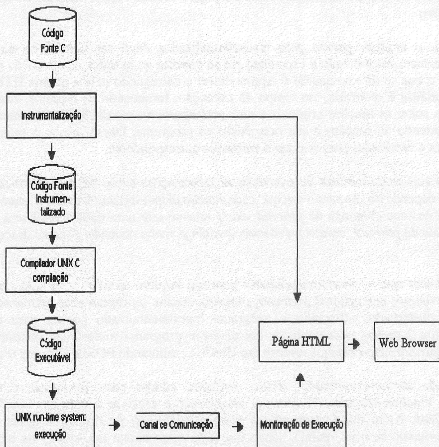
Figura 1 – Fases da animação de um programa multithread
